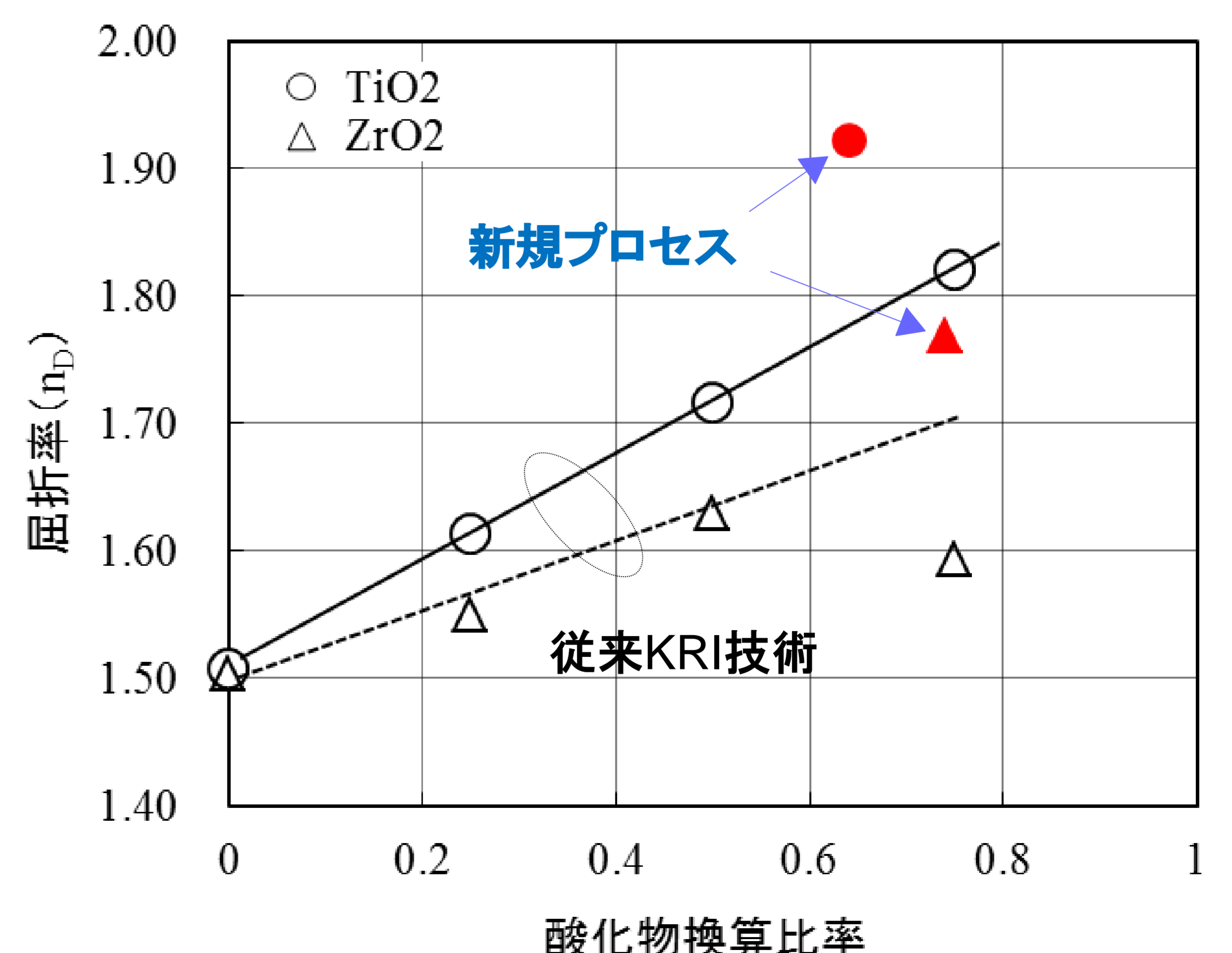
新規ハイブリッド膜の屈折率 (分光反射法測定)
