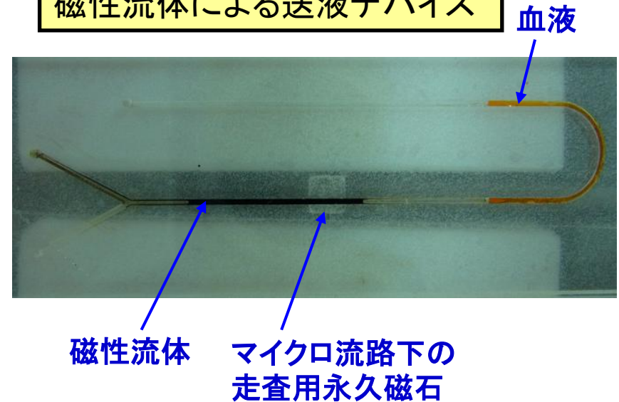
磁性流体による送液デバイス
